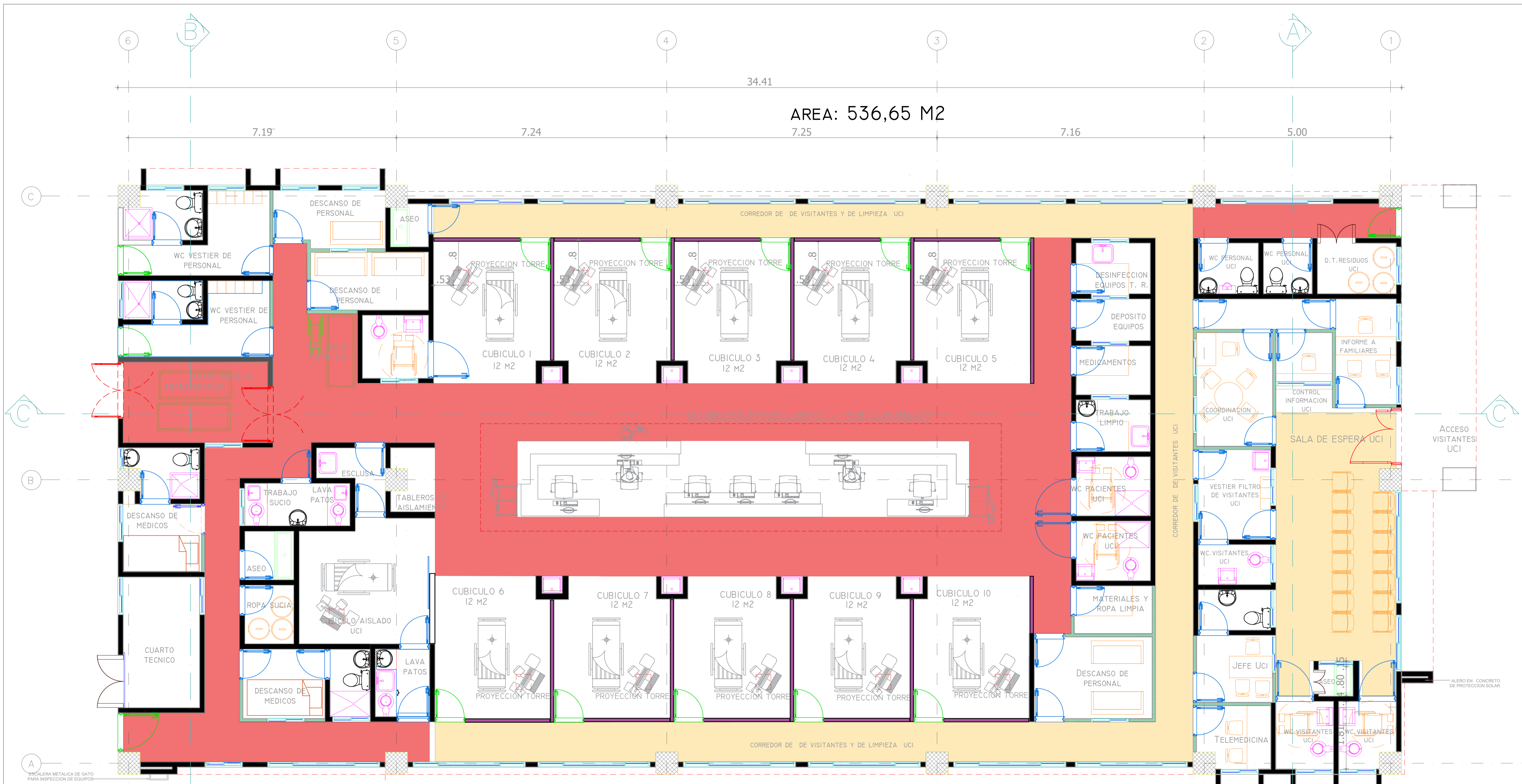
PLANTA ARQUITECTONICA CIRCULACIONES
